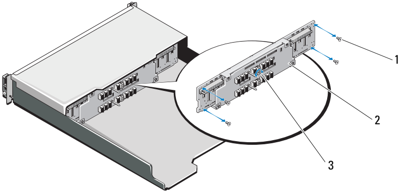
图 16-17. 卸下和安装背板 -PowerVault MD3620f
